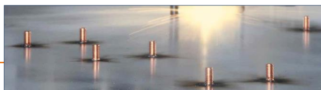
Soudure d'accessoires par décharge de condensateur Discrètes
